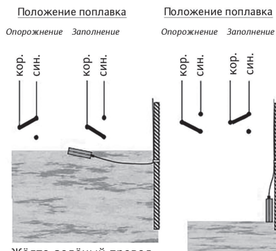
Рис. 6 Электрическое подключение KR 1
